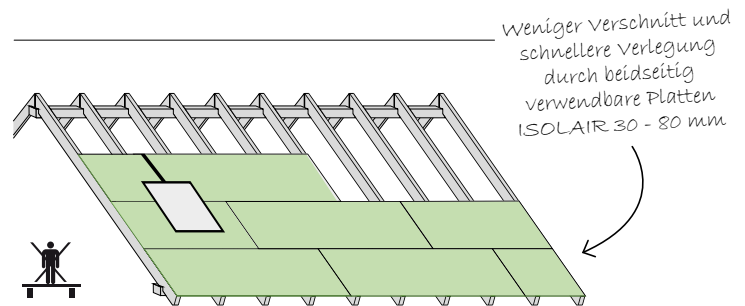
Abb.7 Verlegeprinzip (schematische Darstellung) Platten nur im Sparrenbereich begeben.
