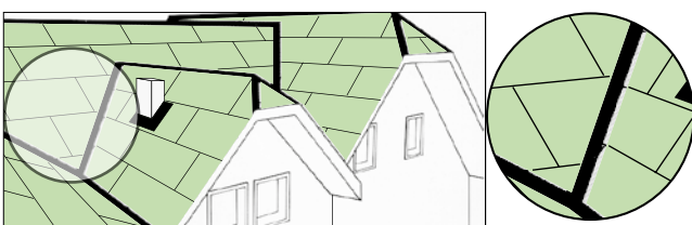
Abb.14 Senkrecht verlaufende Plattenstöße dürfen nicht in Kehlen münden.
