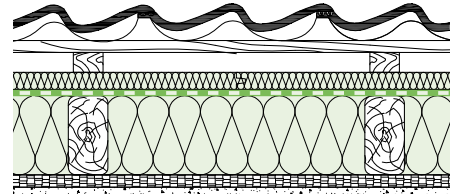
Abb. 16: Konstruktionsbeispiel
