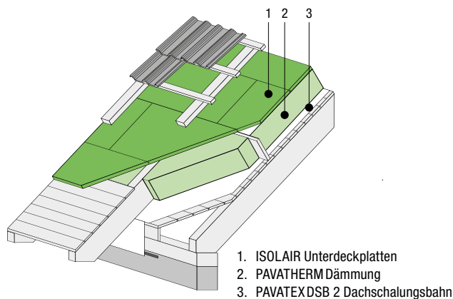
Abb.8 ISOLAIR als Unterdeckung bei einer Aufsparrendämmung
